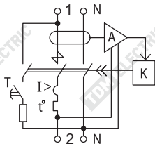
Рисунок 3. Схема подключения
