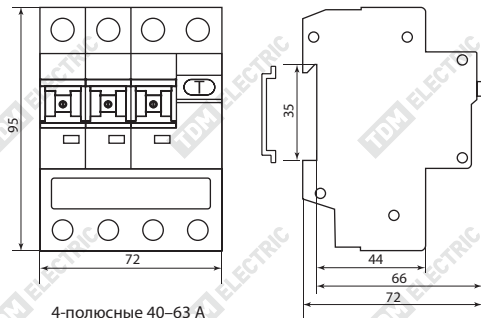
Рисунок 2. Габаритные и установочные размеры, мм
