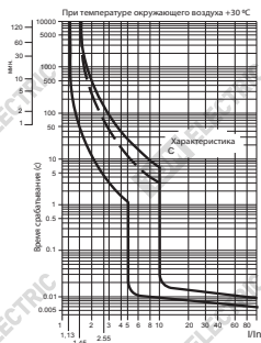
Рисунок 2. Время-токовые характеристики выключателей
