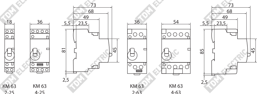
Рисунок 1. Габаритные размеры контакторов, мм
