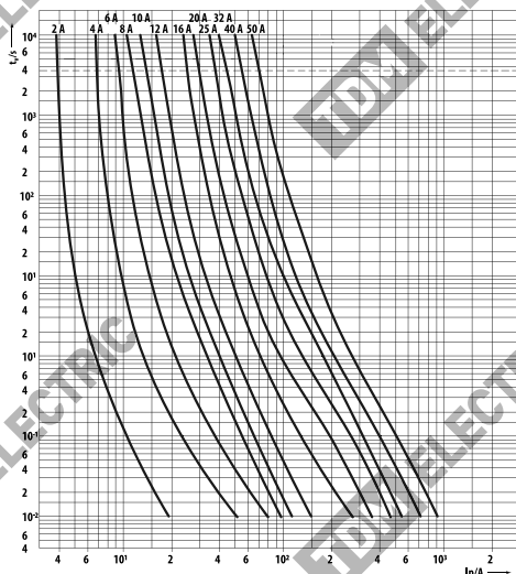
Тип gG, 14x51
