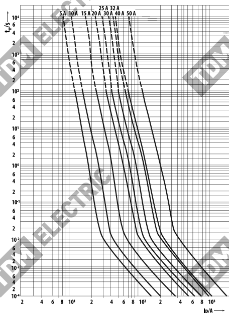
Тип aR, 14x51
