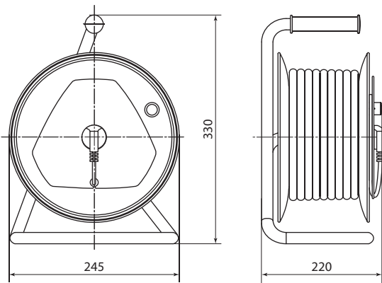
Удлинитель силовой со штепсельным гнездом УК10-001, УК6-001, УК310-001, УК316-001
